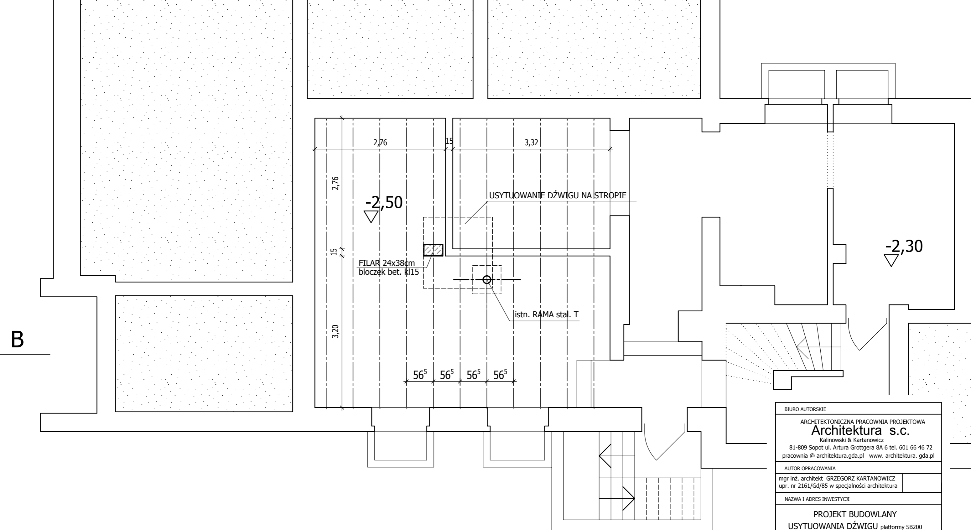
RZUT PODPIWNICZENIA 1:50
